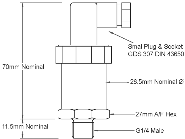
Small Plug & Socket IP65, GDS 307 DIN 43650
